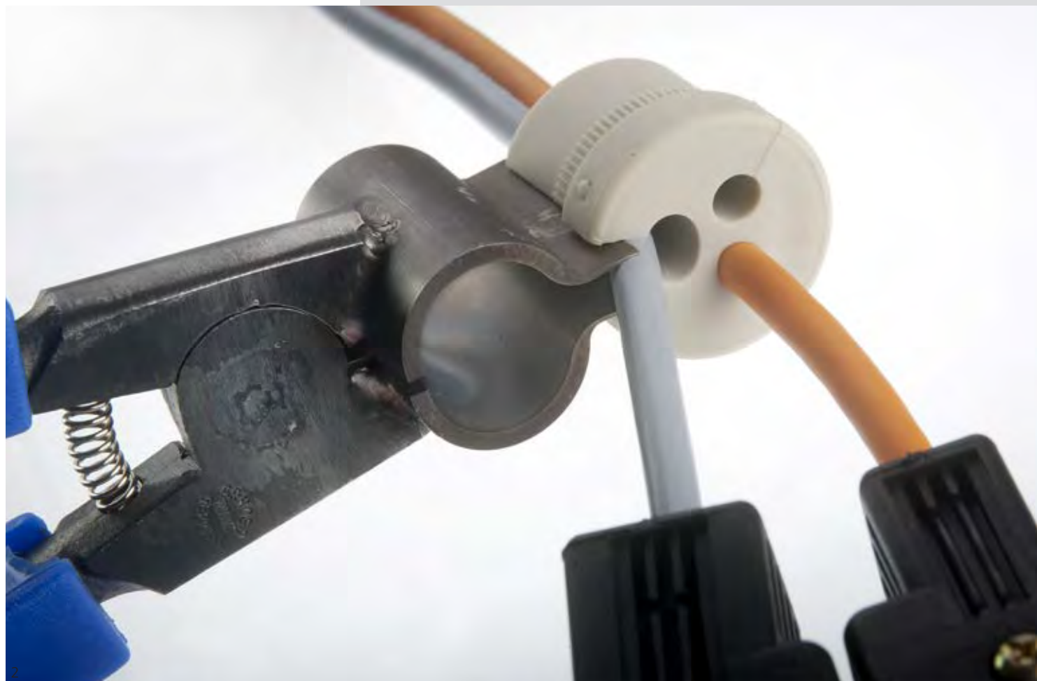
Abb. 1 – UNI FLANSCH in seinen Einzelteilen Fig. 1 – Individual components of the UNI Flange®
